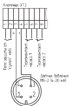
Рис. 1 Пример подключения датчика давления МН-2 WIKA
